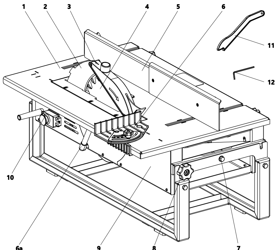
Рисунок 1. Общий вид станка в режиме пиления
