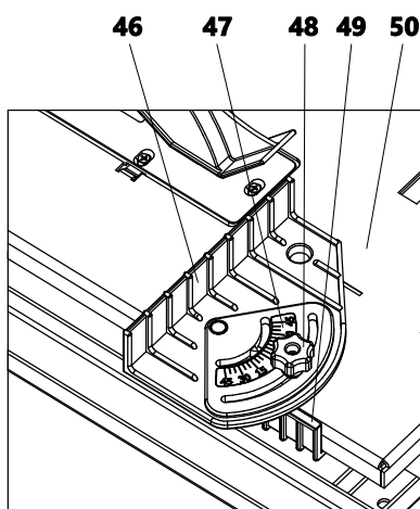
Рисунок 10. Приспособления для поперечной распиловки под углом
