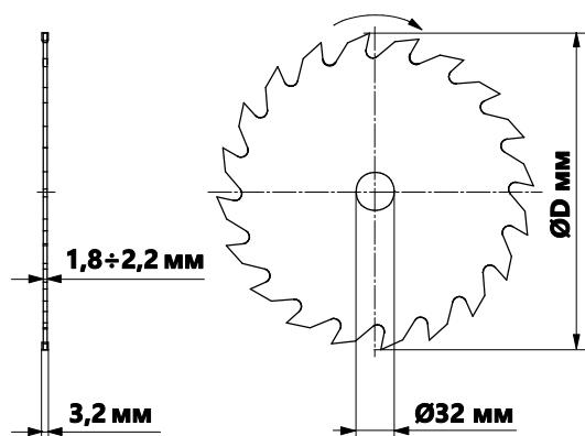
Рисунок 16. Диск пильный
