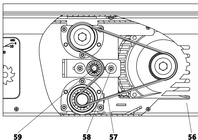
Рисунок 17. Установка приводного ремня
