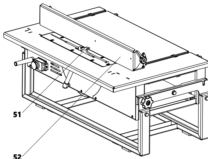
Рисунок 11. Общий вид станка в режиме фрезерования дисковой фрезой 51 – фреза дисковая, 52 – линейка
